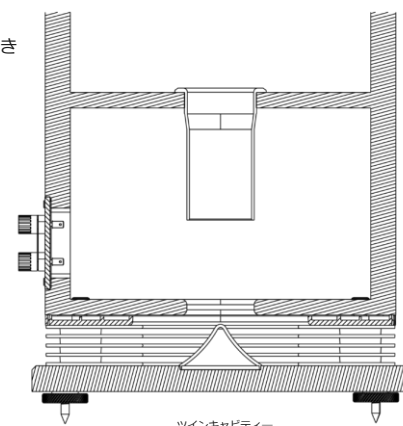
ツインキャビティ
