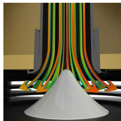
低域ポートの波面を 360°変換
